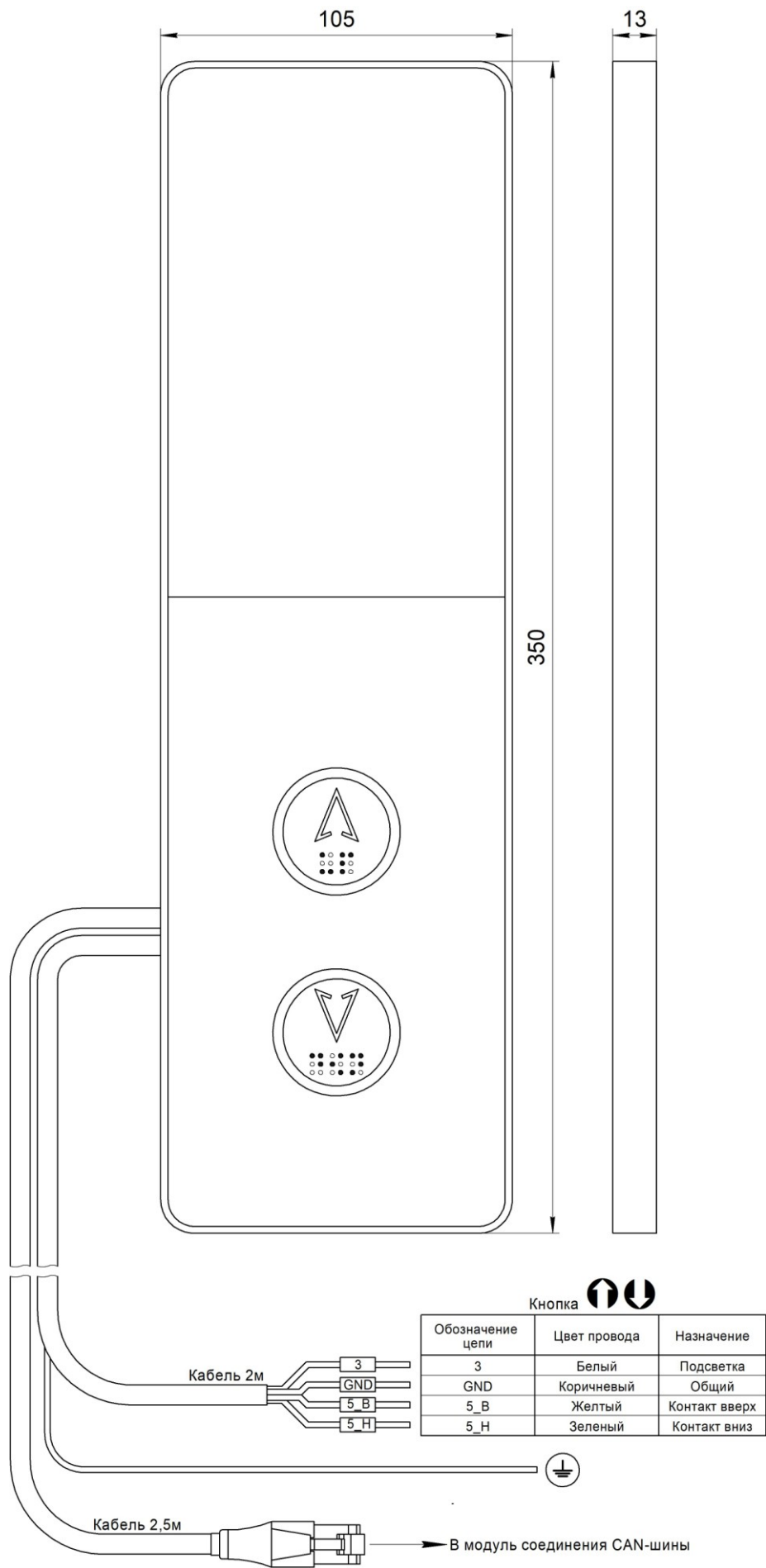
Рис.1 Внешний вид, габаритные и установочные размеры Вызывного поста МАЛАХИТ (жгут RJ45) НШЕК.468381.016
